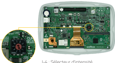
I-4 : Sélecteur d'intensité
