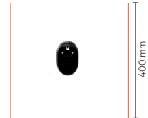
I-2.2: Håll avståndet runt hållare för fordonsladdningskontakt
