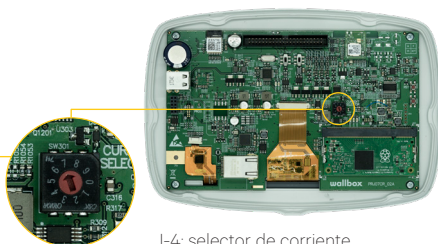
I-4: selector de corriente
