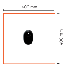
I-2.2: Abstand um die Halterung für Ladestecker
