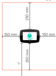
I-2.1: Area di montaggio
