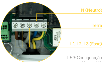
I-5.2: Configuração monofásica (1P)
