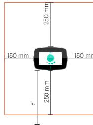
I-2.1 : Surface de montage
