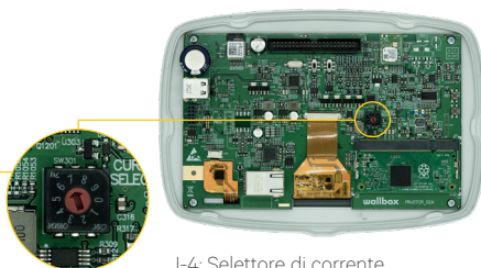
I-4: Selettore di corrente
