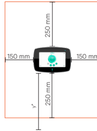
I-2.1: Zona de montaje
