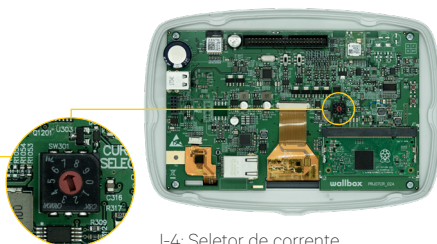
I-4: Seletor de corrente
